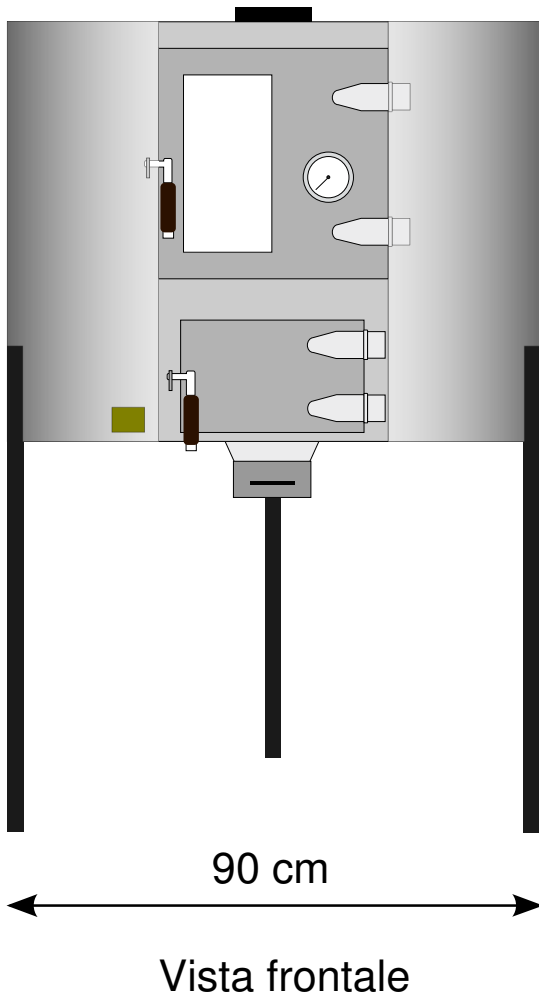
Forno SAF mod. 90 rinforzato
